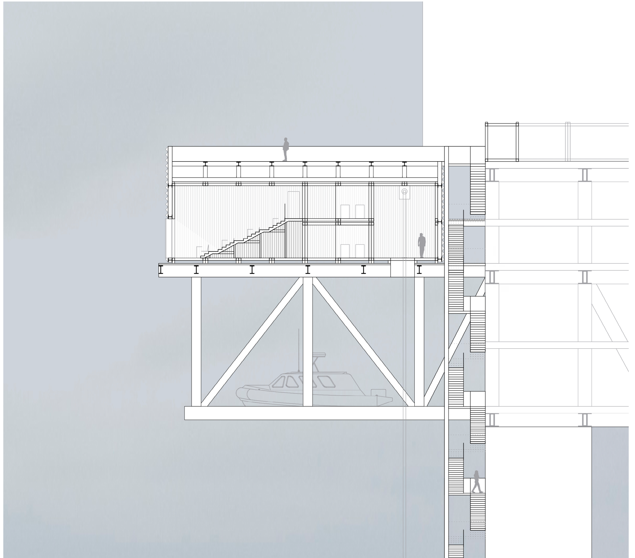
SCHNITT EE 1:200
