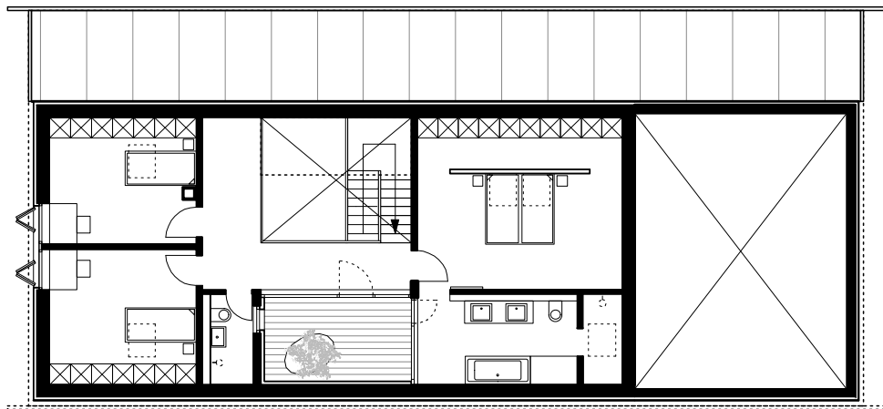
GRUNDRISS DG 1:200
