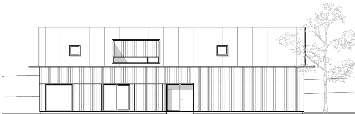
ANSICHT OST 1:200
