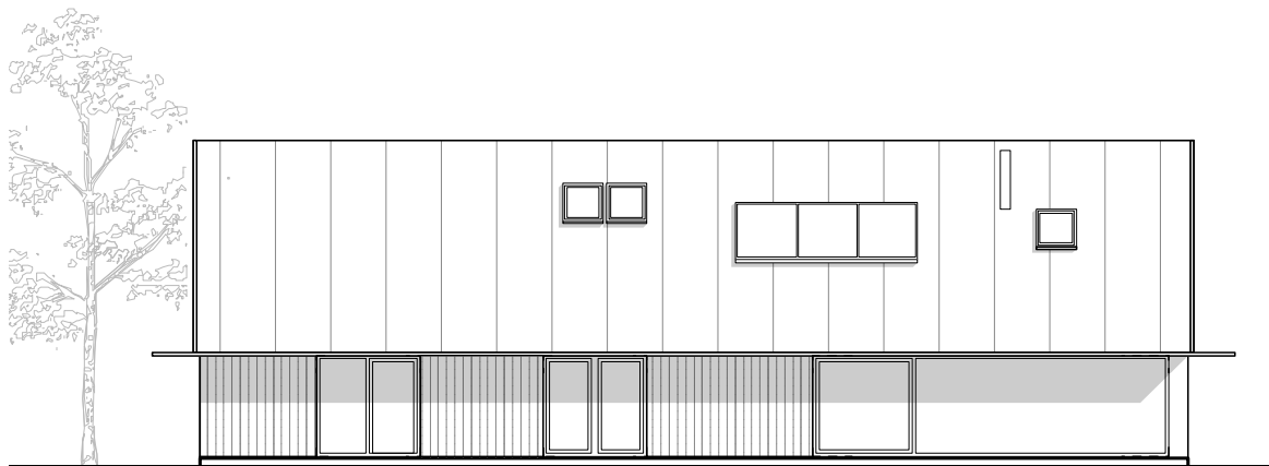
ANSICHT WEST 1:200
