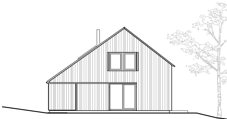
ANSICHT SÜD 1:200
