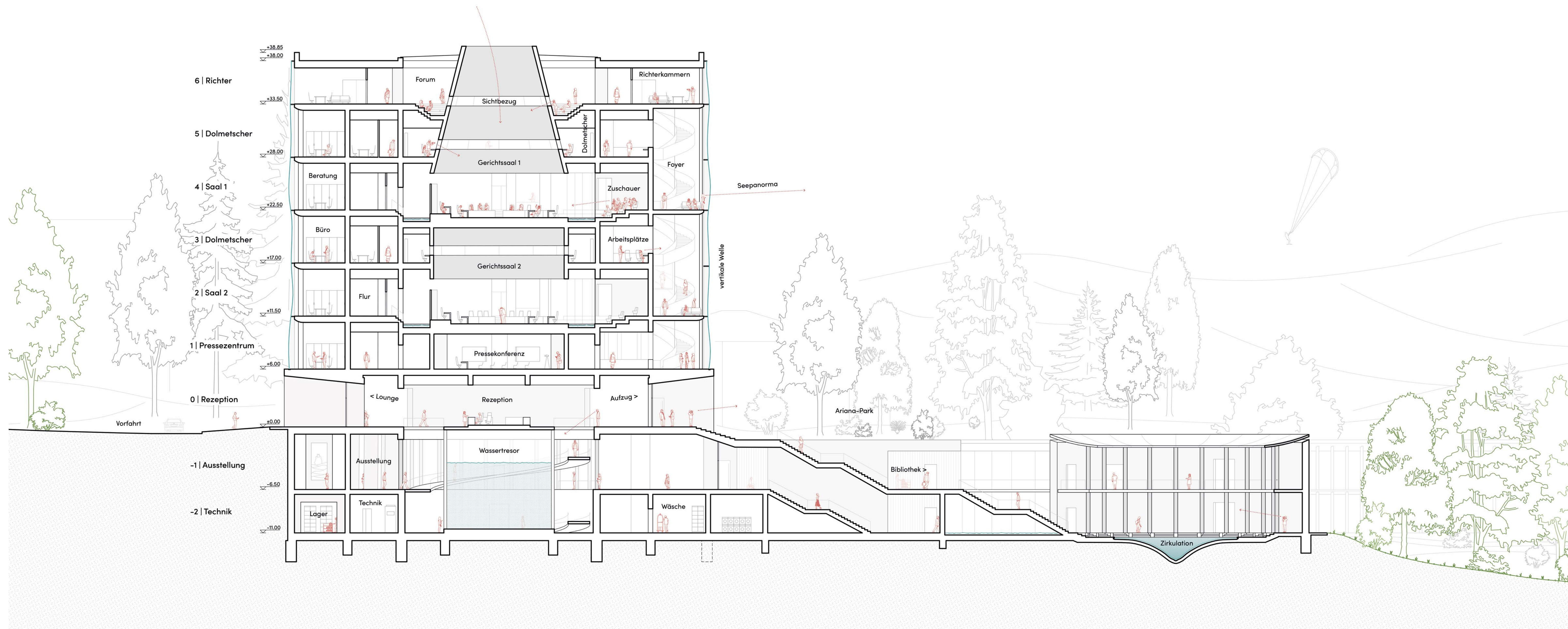
Schnitt C | 1:200 Eingebettet in der Topografie
