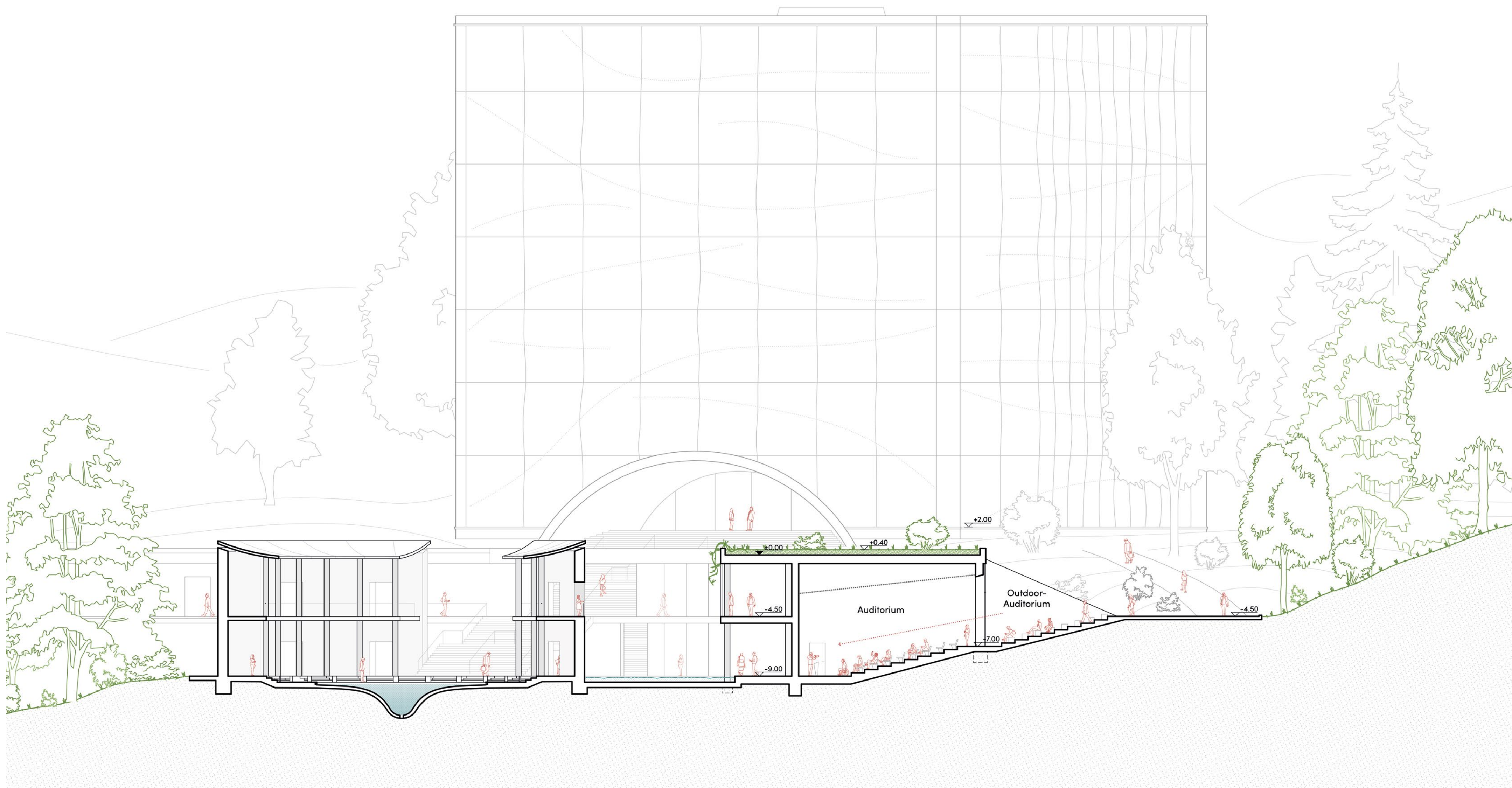
Schnitt E | 1:200 Erweiterung des Auditoriums in den Außenbereich
