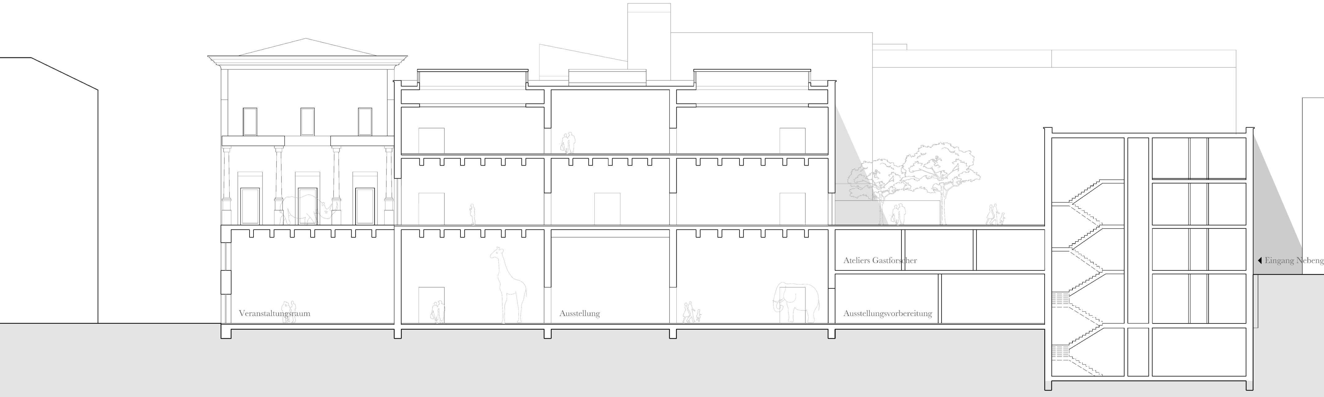
SCHNITT A-A | 1:200
