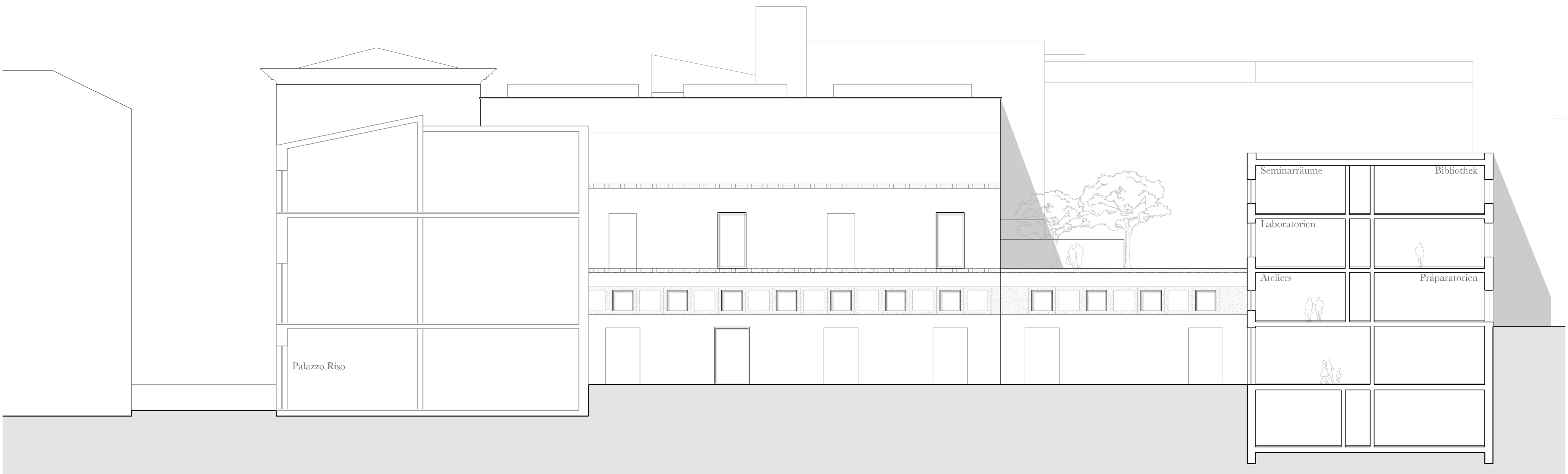
ANSICHT OST | 1:200
