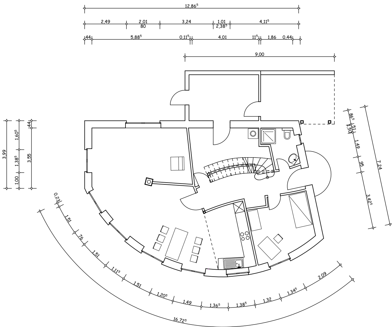
Erdgeschoss
