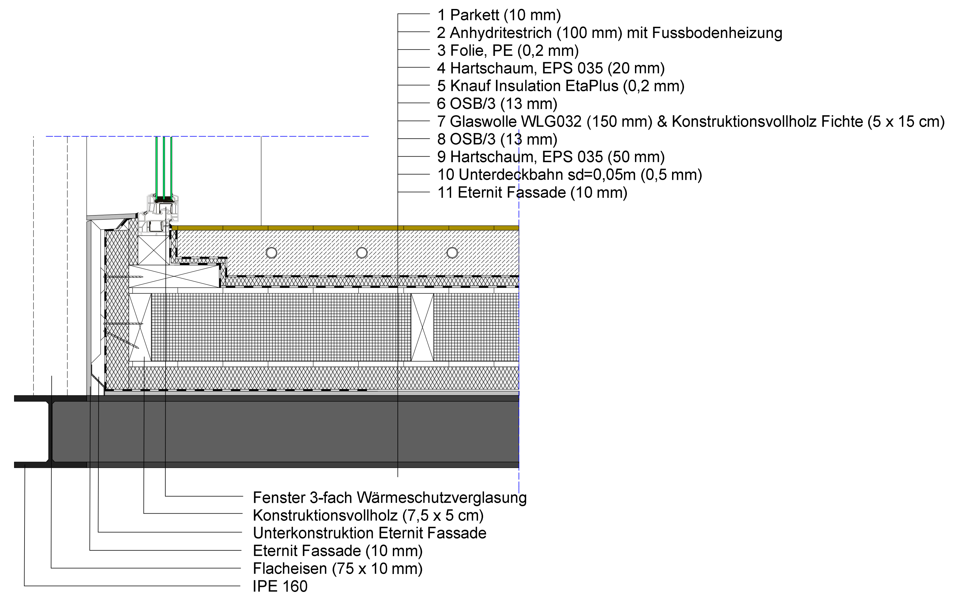
Detail 04: Wand-Boden Anschluss mit Fenster
