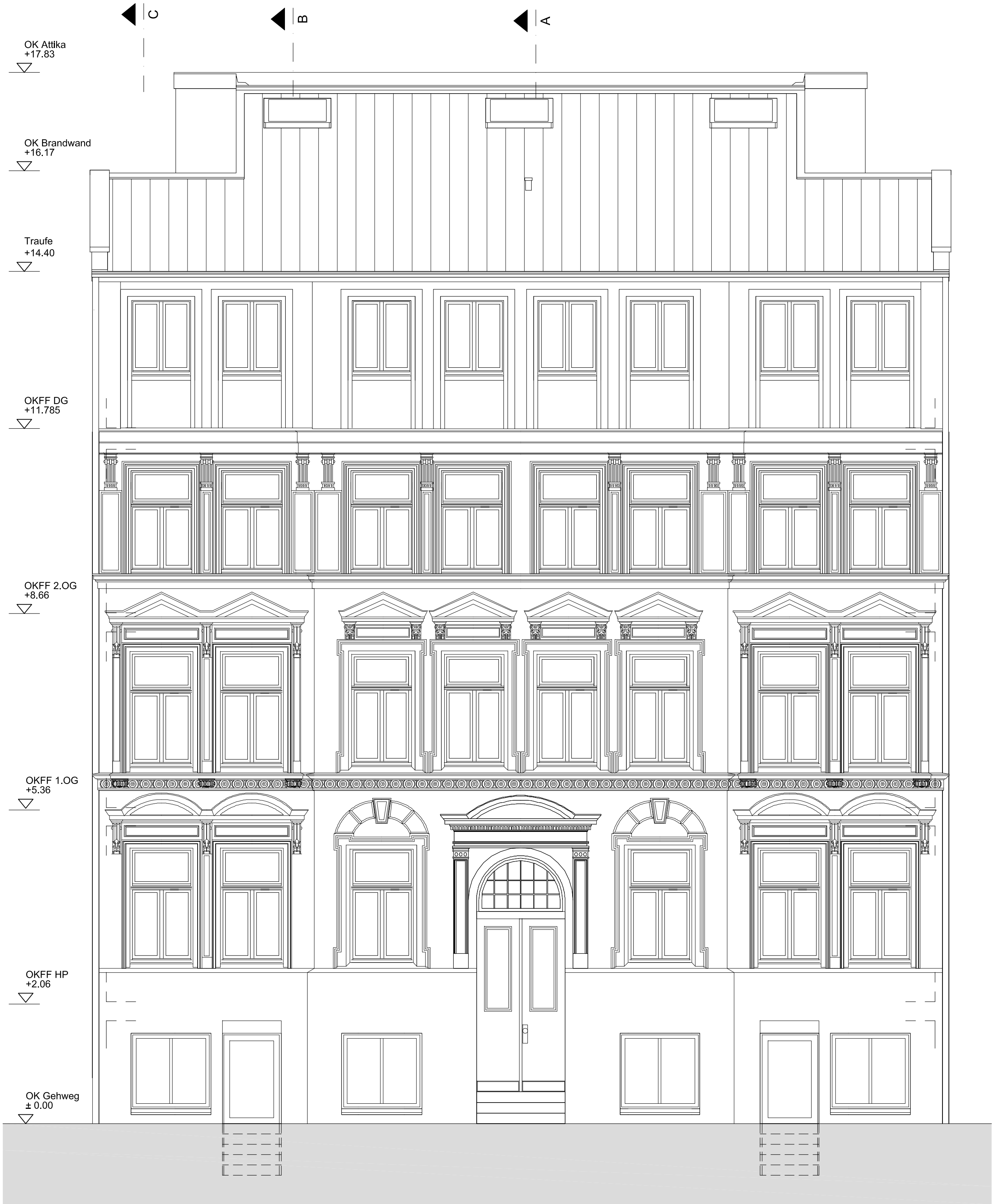
Ansicht Westen (1:50)
