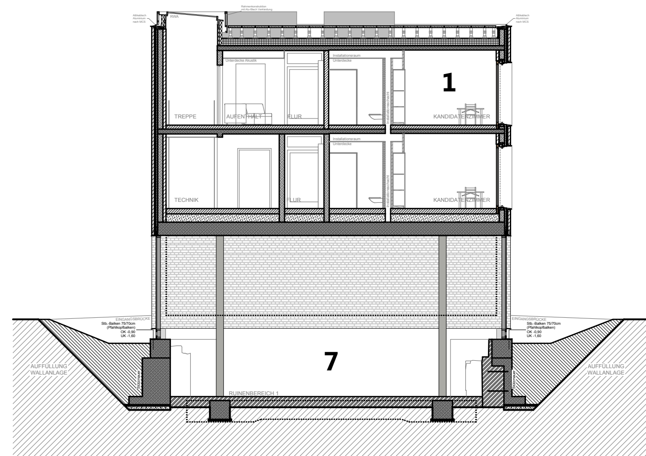
Querschnitt Bauteil 1
