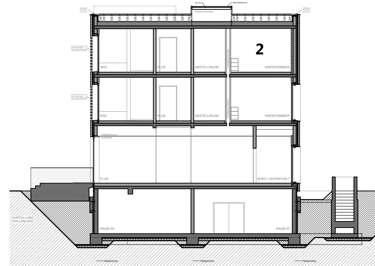
Querschnitt Bauteil 2
