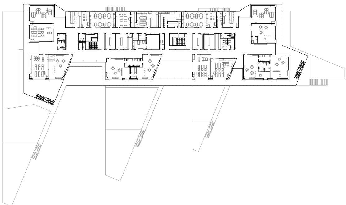
GRUNDRISS 2. OBERGESCHOSS
