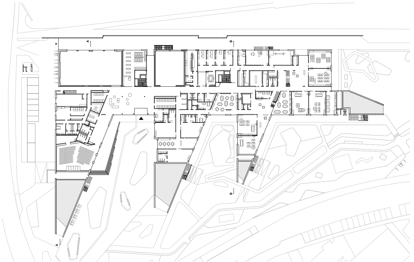
GRUNDRISS ERDGESCHOSS
