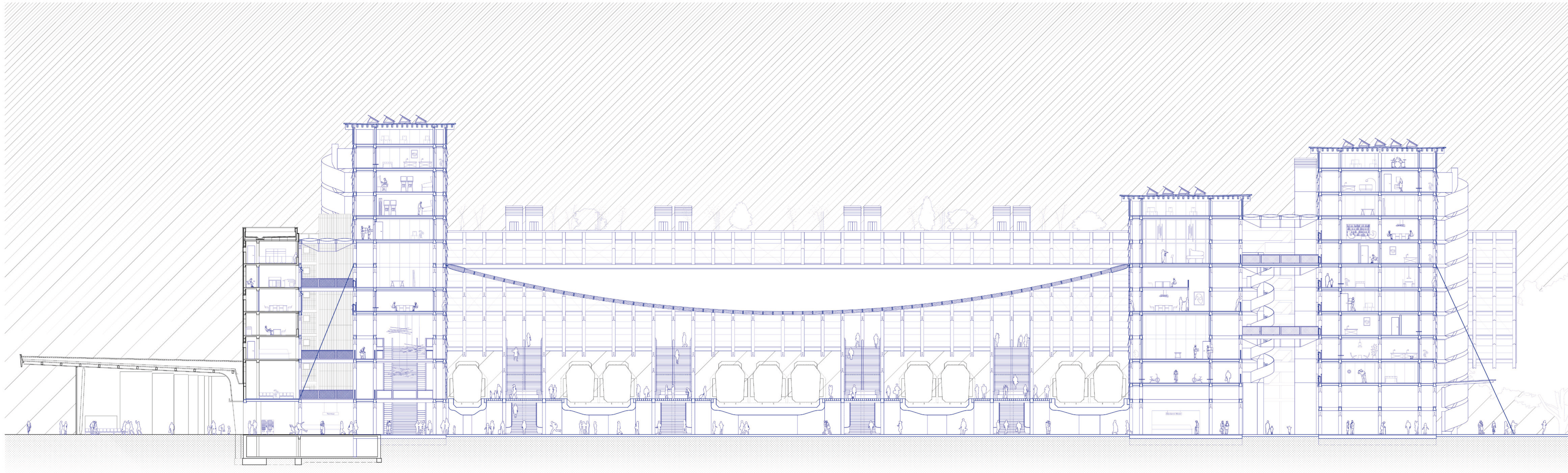
Querschnitt A-A M 1:200 Die Brücke verbindet alle Gebäudeteile miteinander und ermöglicht den Austausch zwischen Reisenden und Nutzenden. Der große Bruder und die Zwillinge werden zur raumhaltigen Wand der Bahnhofshalle.
