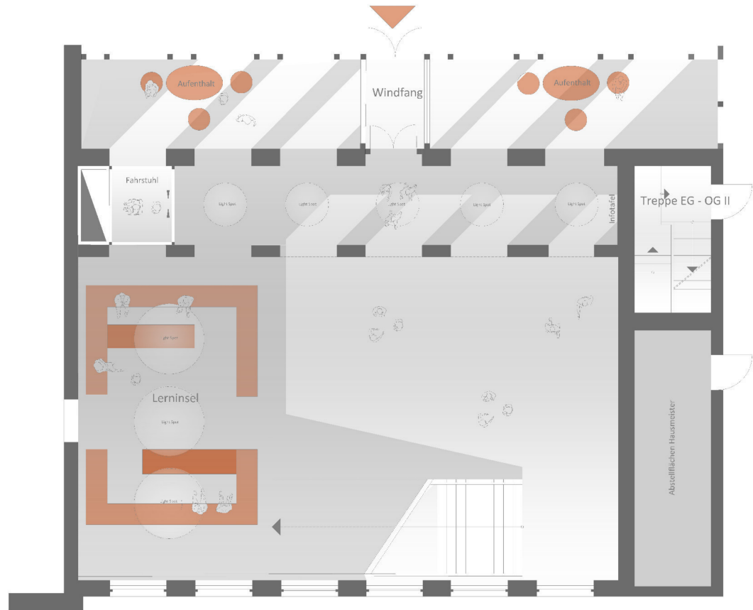
Grundriss EG - Foyer Nordflügel - M. 1:50
