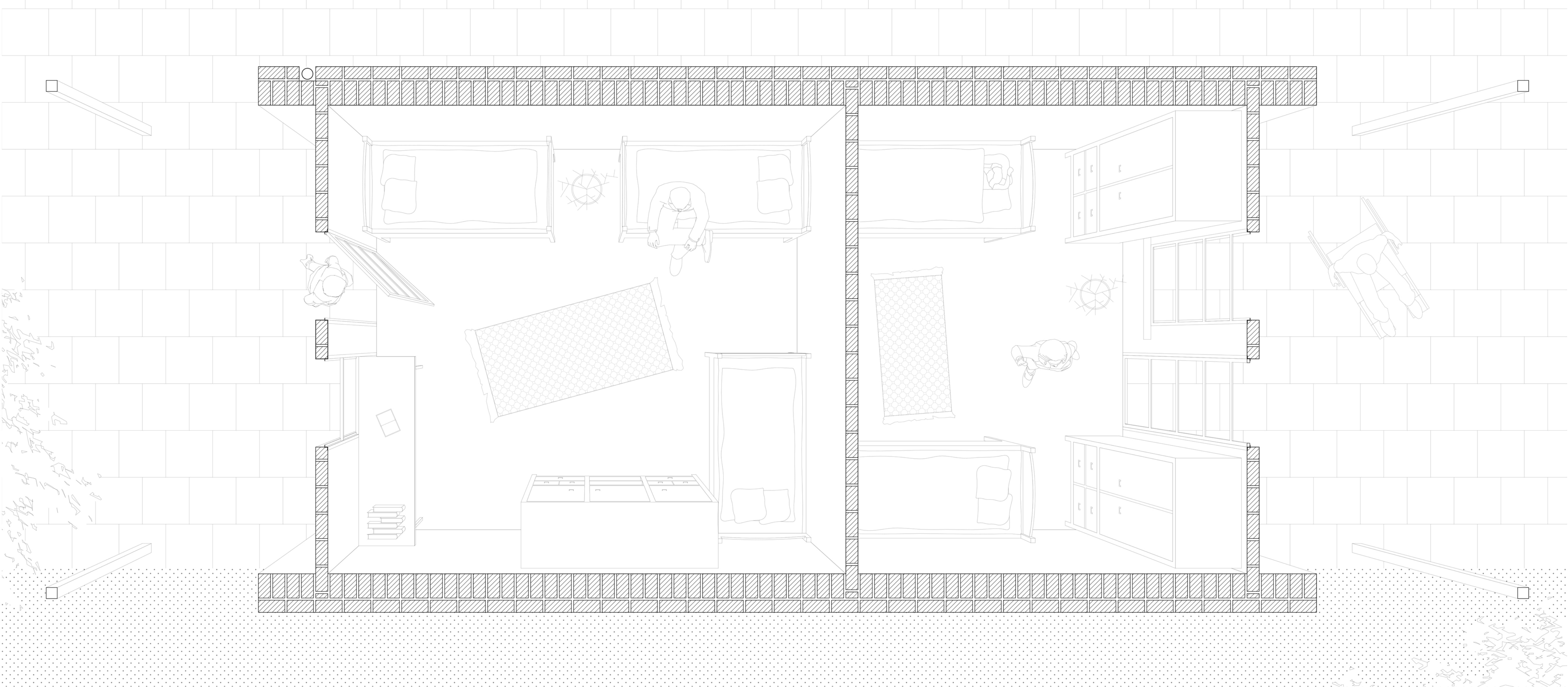
Detailgrundriss | M 1:20
