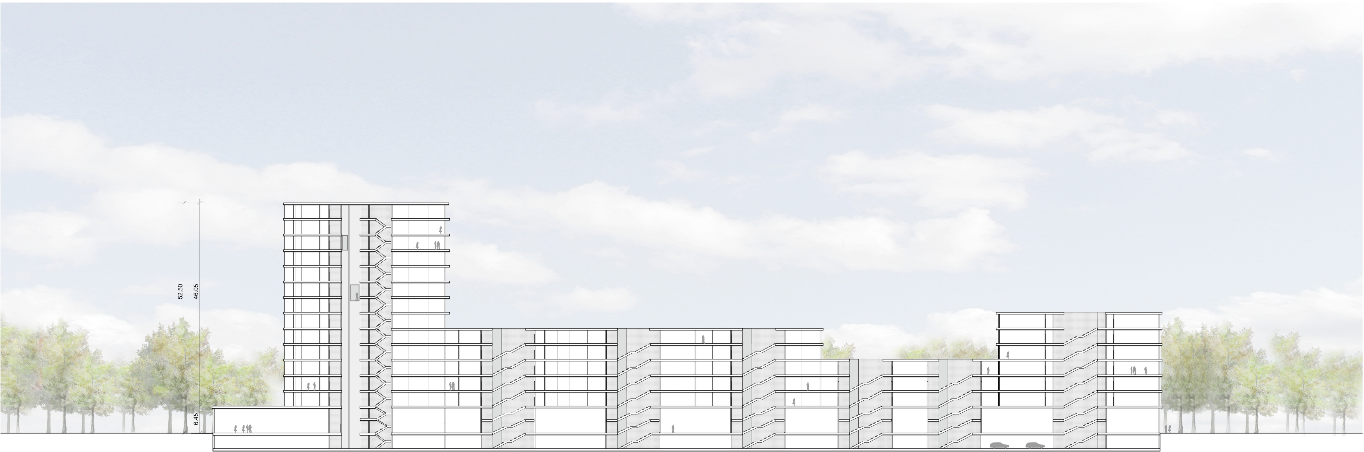
LÄNGSSCHNITT A-A 1:500
