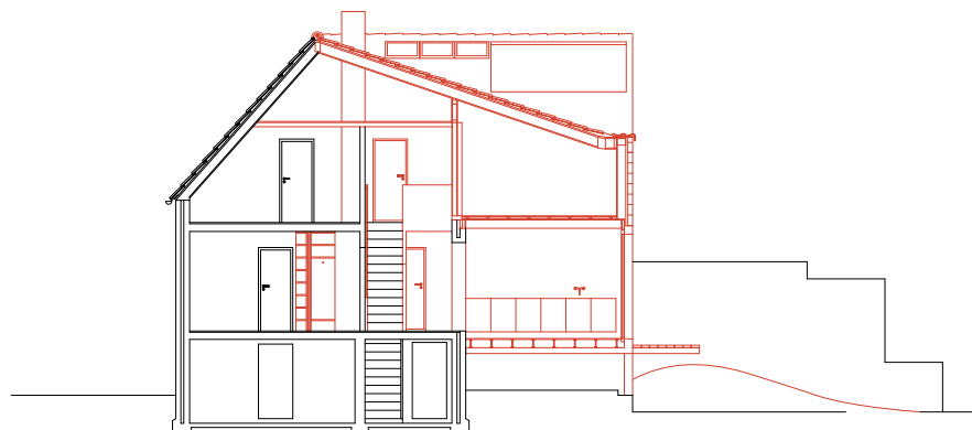
Schnitt D-D/ Section D-D
