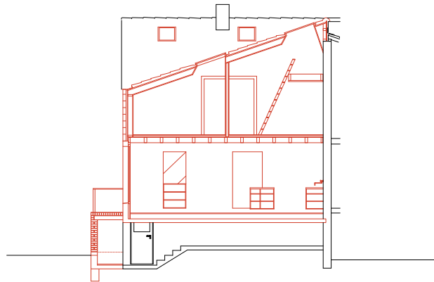
Schnitt B-B/ Section B-B
