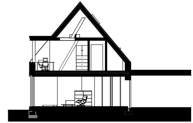
S-05 Schnitt Ost 3 1:200
