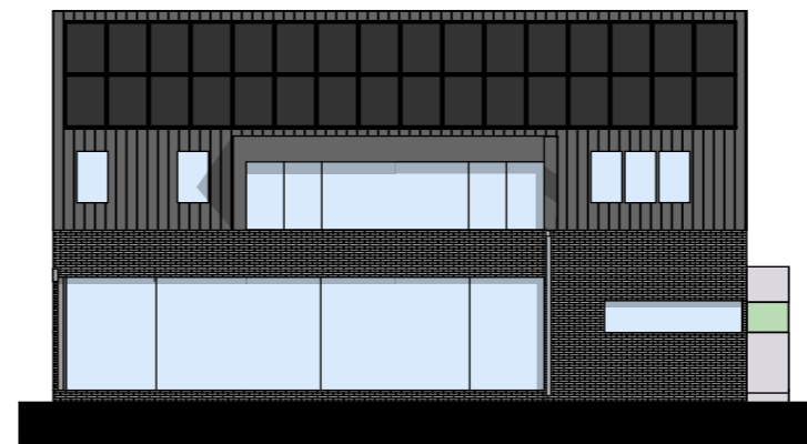
A-02 Süd KAP12 Ansicht Süd KAP12 1:200
