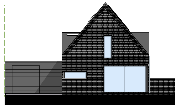
A-03 West Ansicht West 1:200
