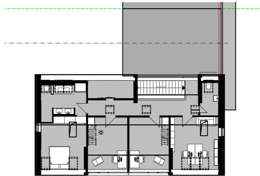
1. 1.OG 1:200
