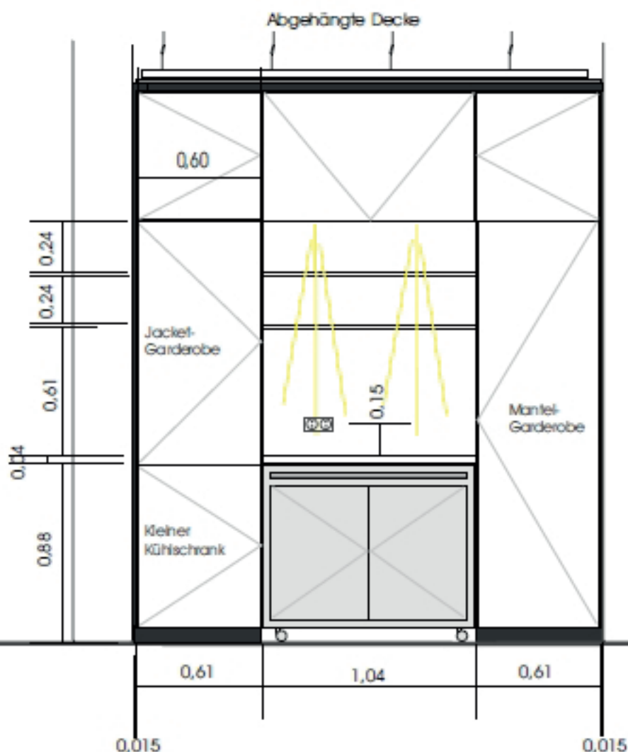
Ansicht M 1:30
