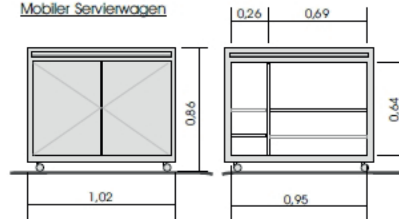
Ansicht M 1:30
