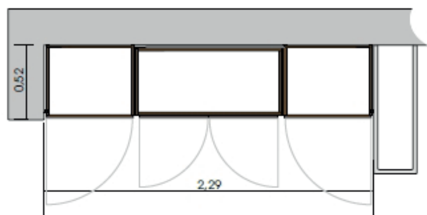
Horizontalschnitt M 1:30
