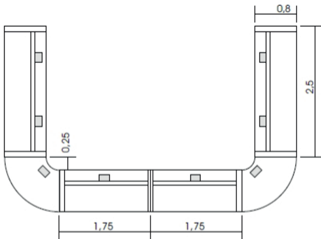
Grundriss Konferenztisch-Module M 1:50
