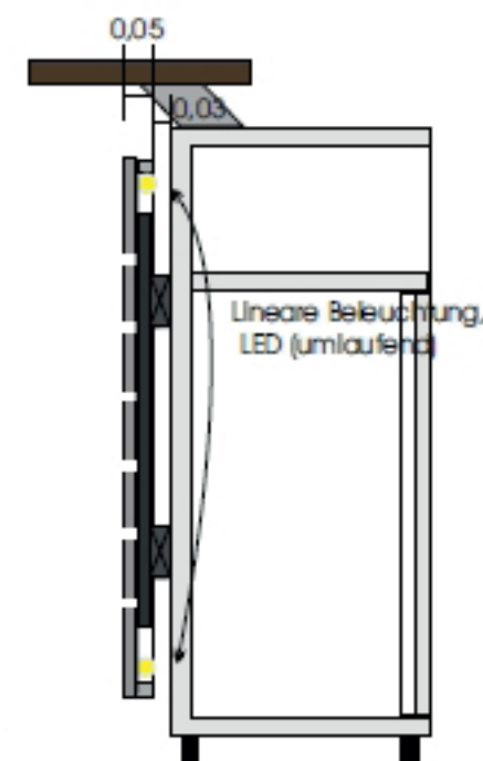
Detail D-D M1:15
