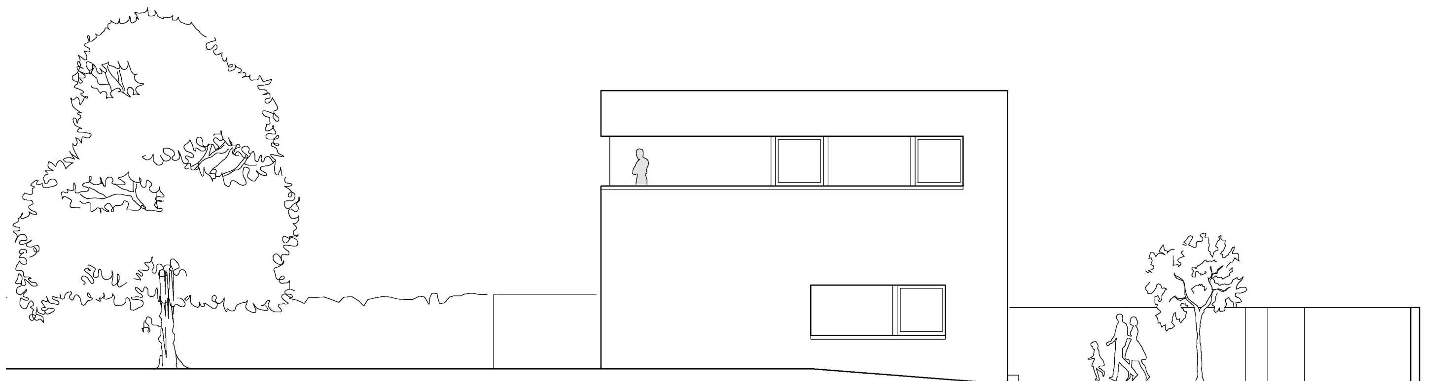
Ansicht Ost
