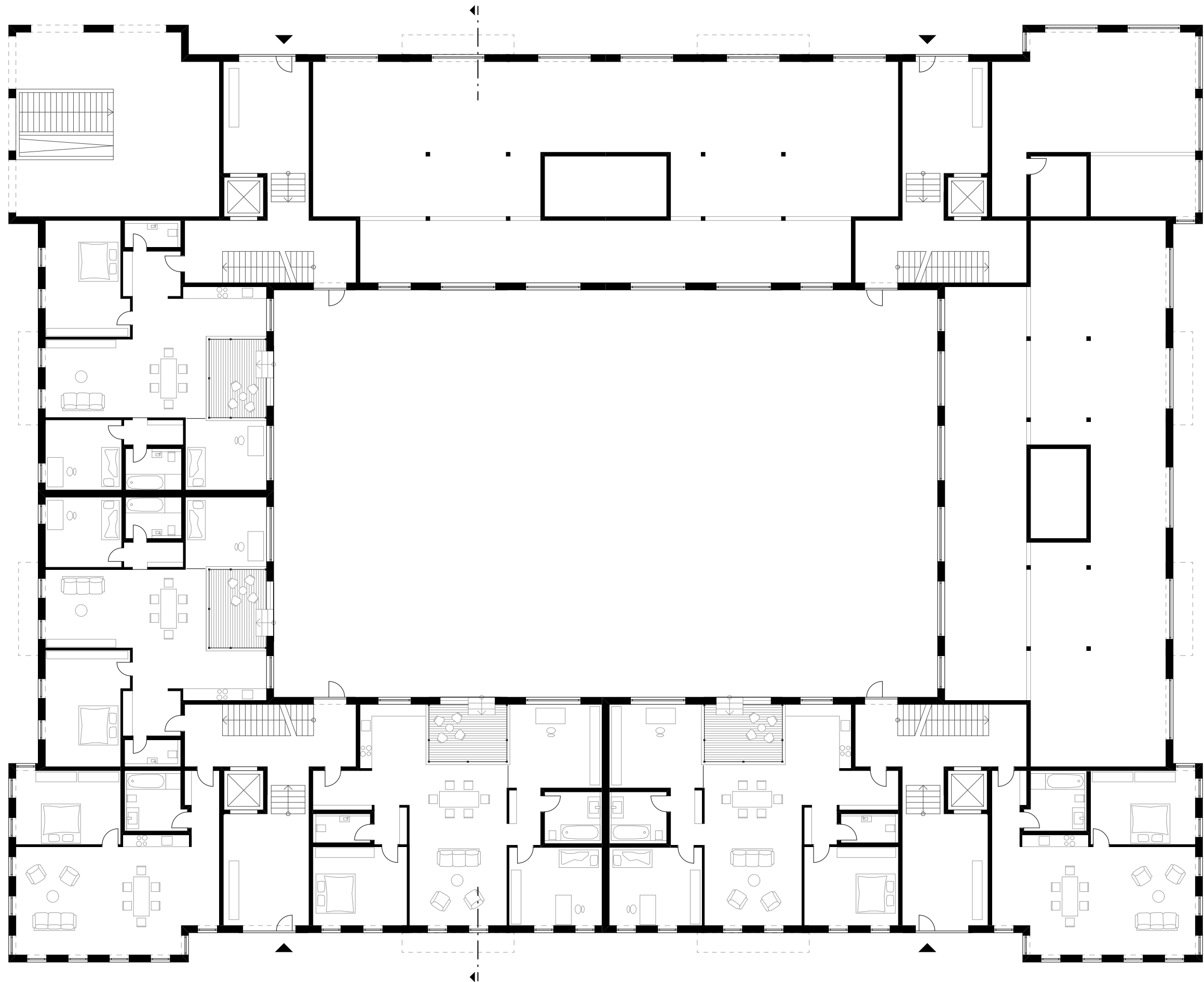
Grundriss Erdgeschoss
