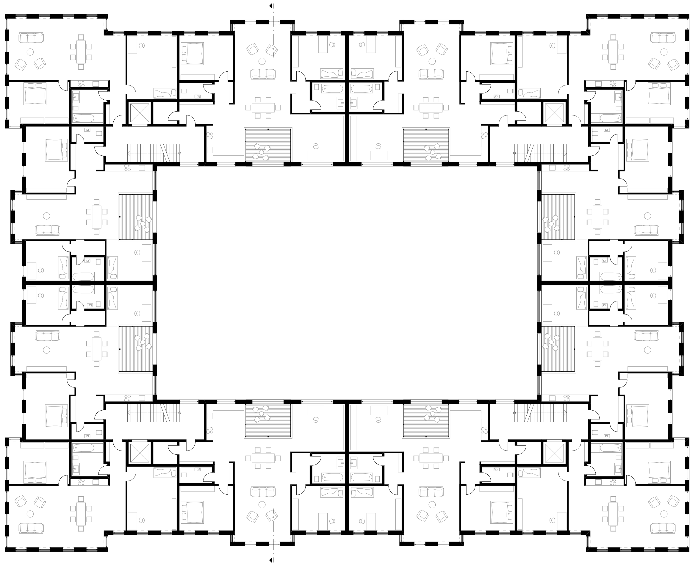
Grundriss Regelgeschoss
