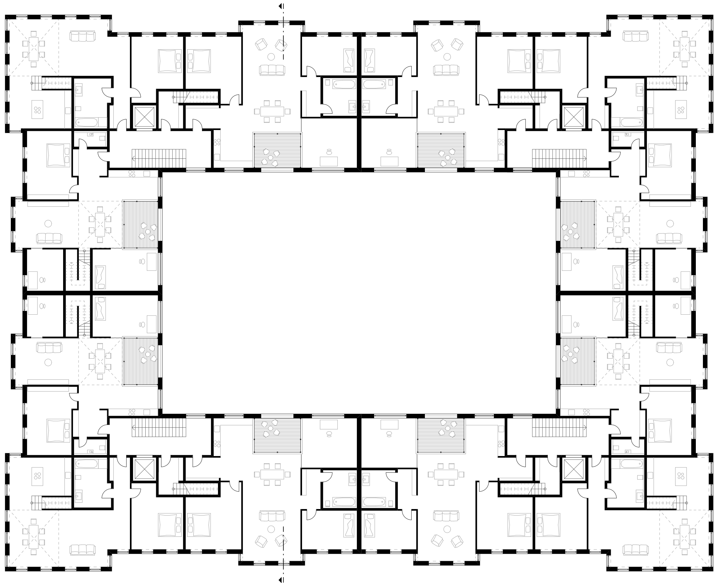
Grundriss 4.OG
