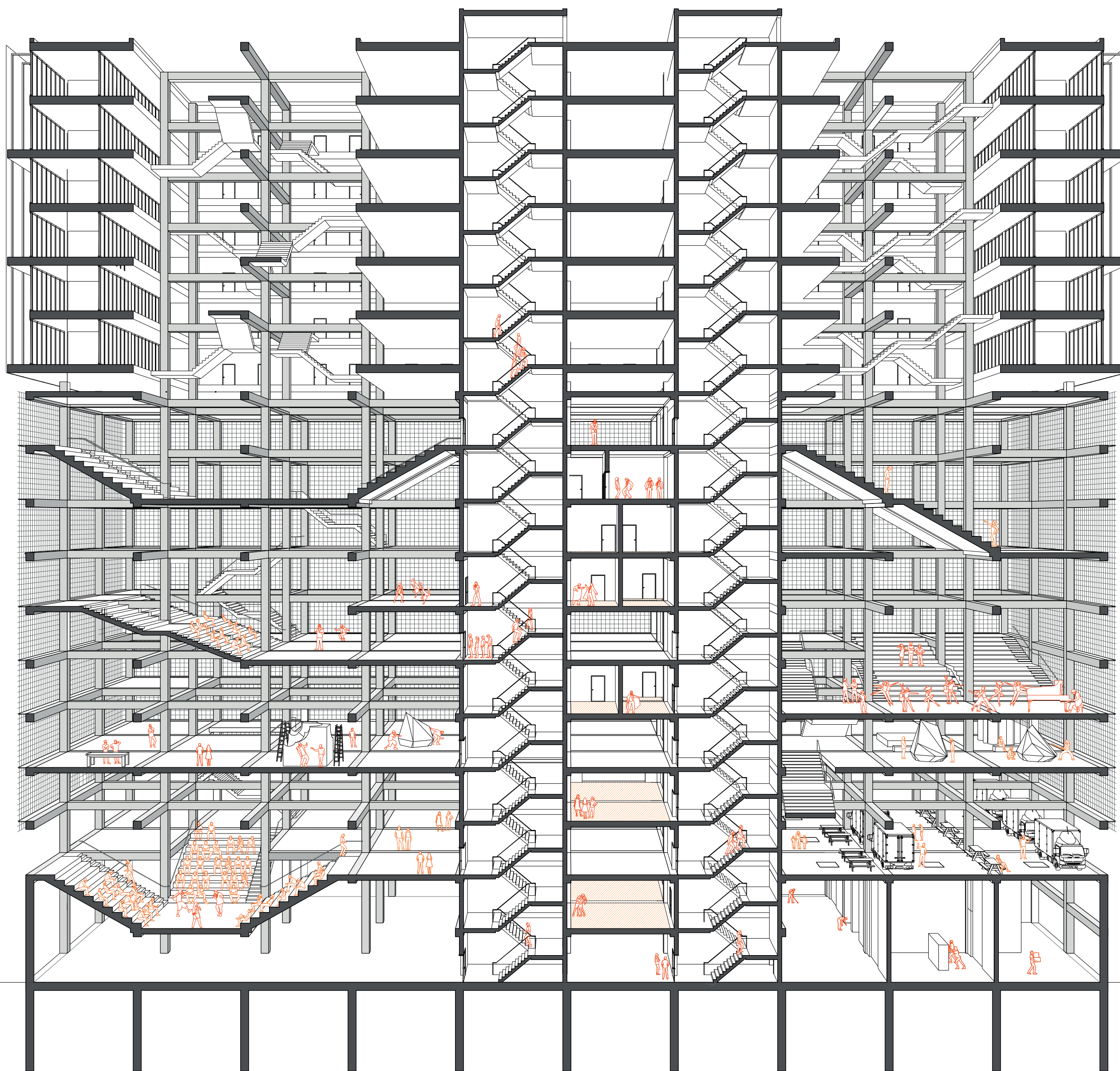
Schnitt A - A M 1:250
