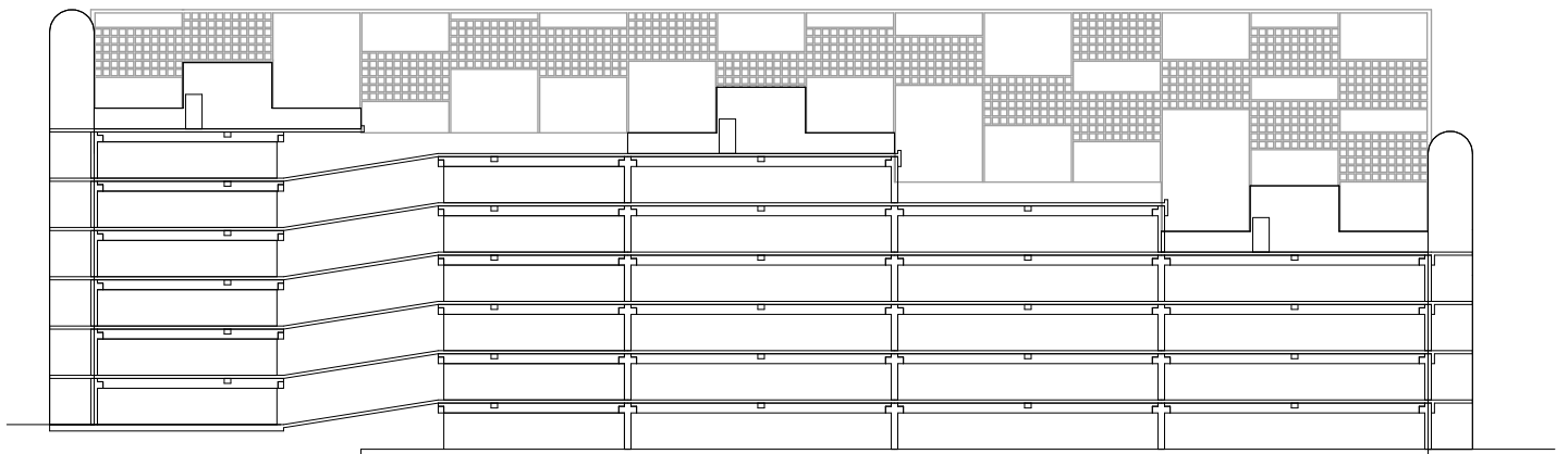
Längsschnitt
