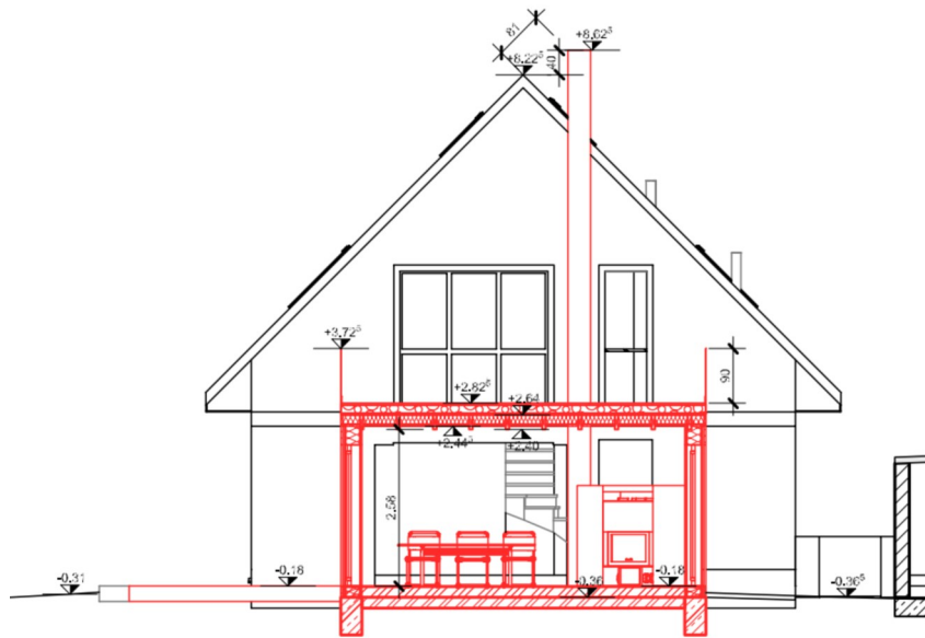
Schnitt C-C
