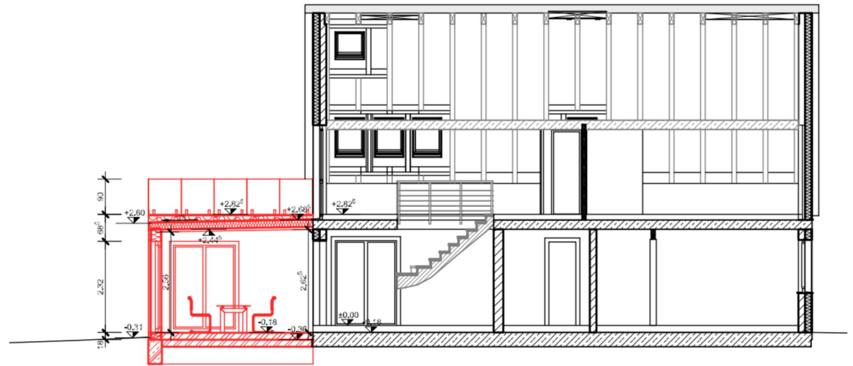
Schnitt D-D
