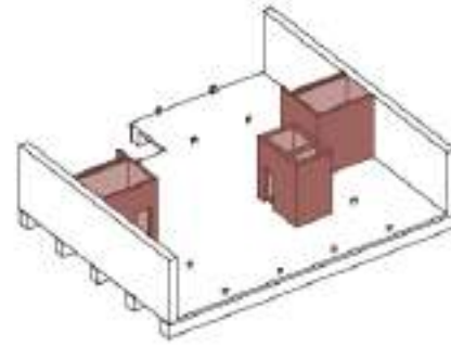
3. Aussteifende Massivholz Kerne
