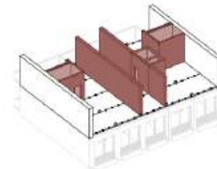
2. Aussteifende Massivholz Kerne + Stiegenhauswände
