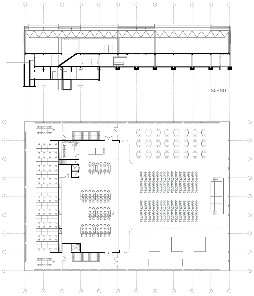
OBERGESCHOSS
