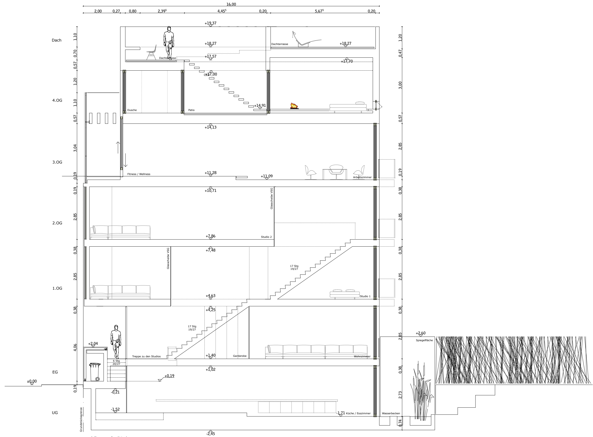
Längsschnitt 1
