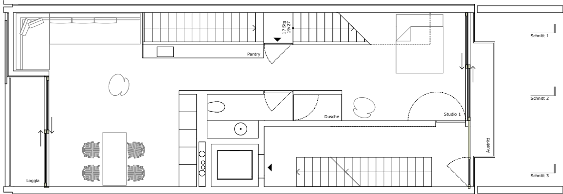
1. OG
