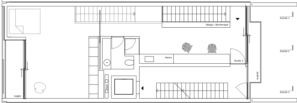
2. OG
