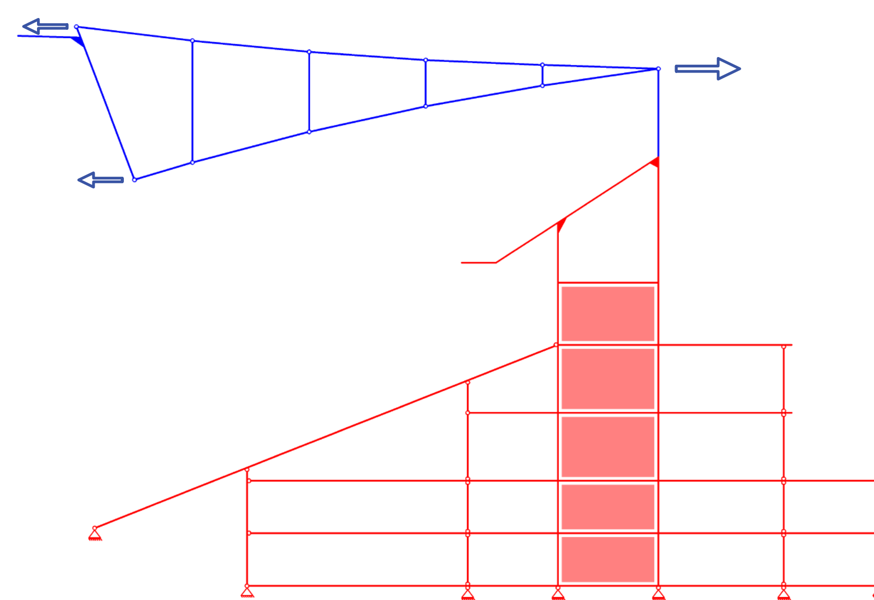
Schnitt Statisches System Maßstab 1:200
