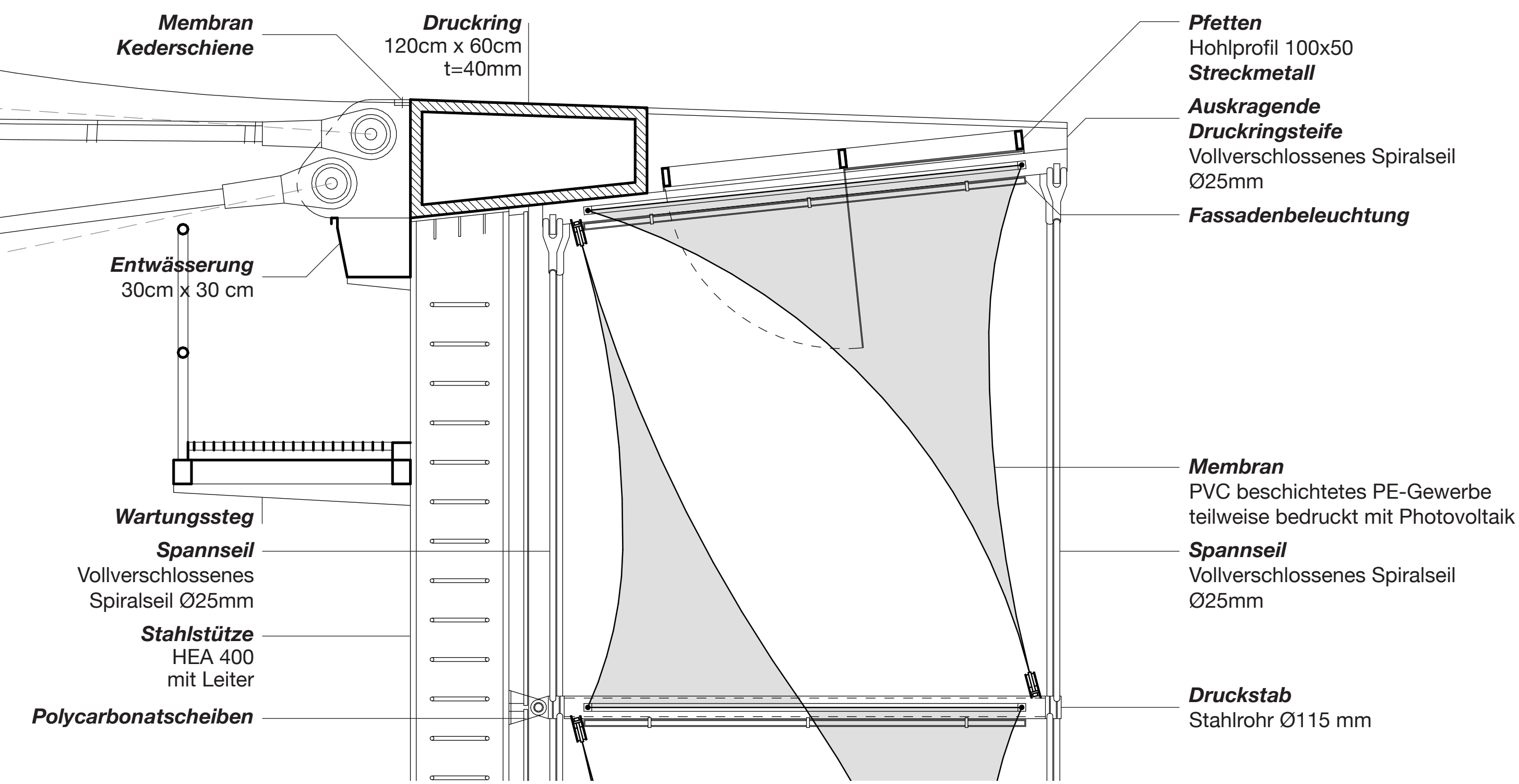
Druckringdetail Maßstab 1:20
