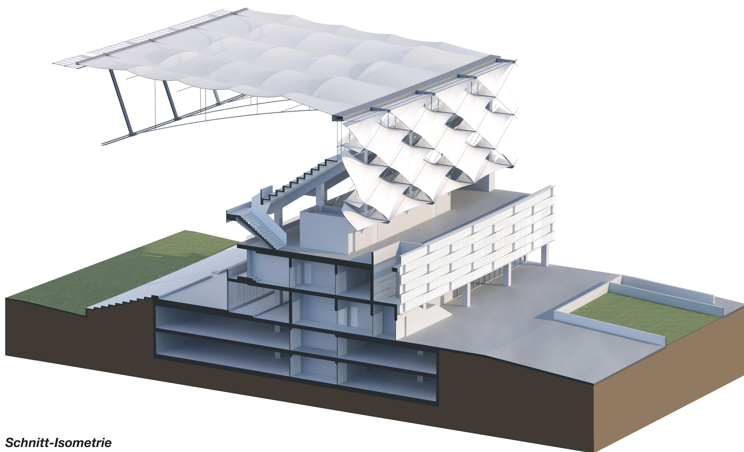
Schnitt-Isometrie
