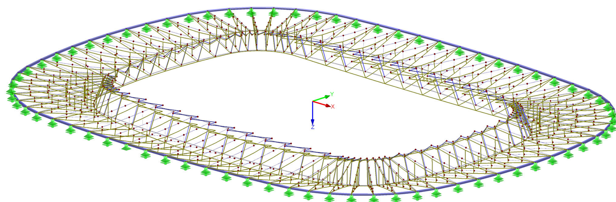
Globale Verformungen
