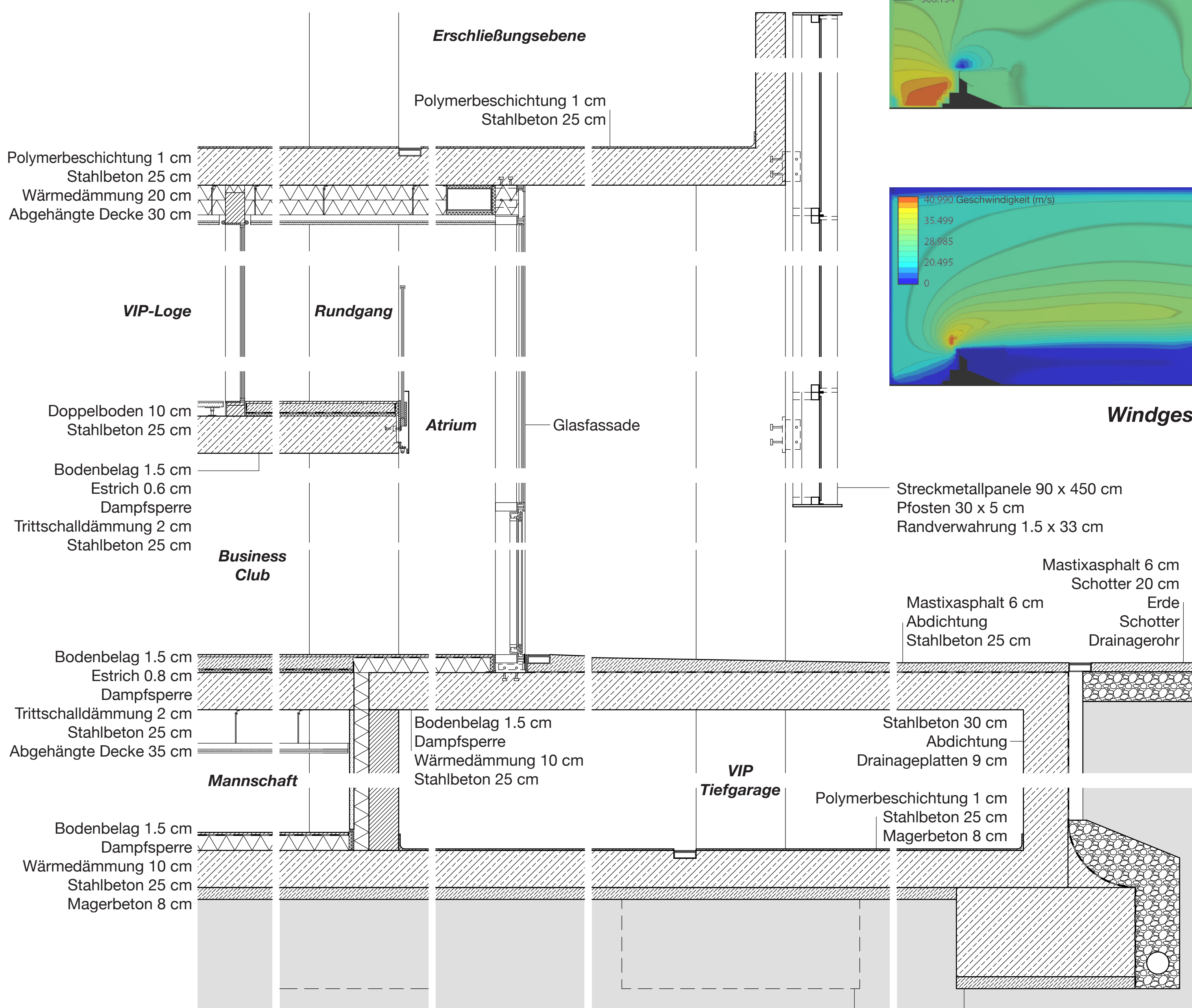
Fassadenschnitt C-C Maßstab 1:20
