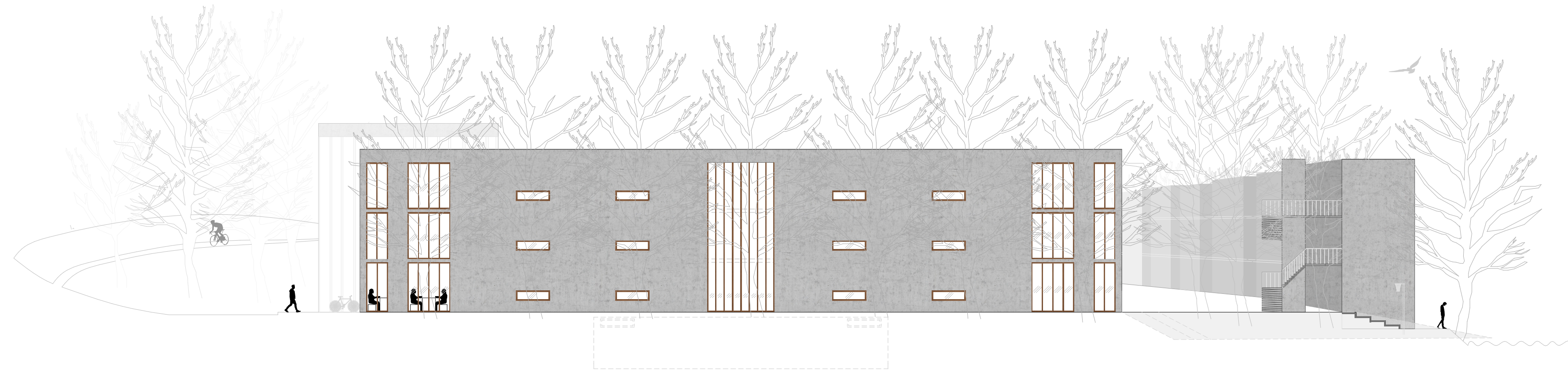
ANSICHT NORD BIBLIOTHEK/VERWALTUNG_M1.200
