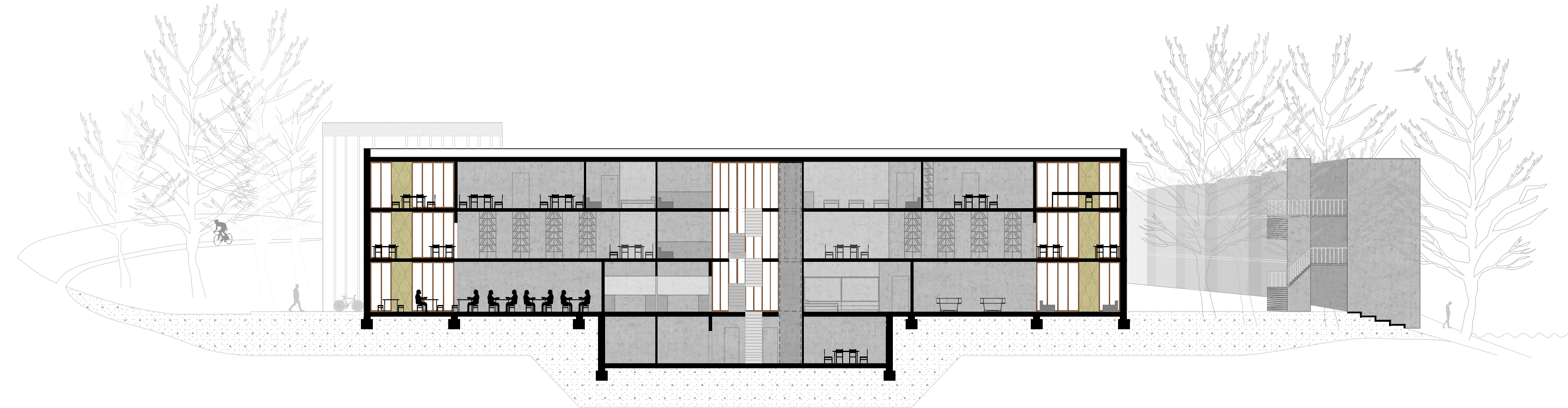
SCHNITT B-B_M1.200
