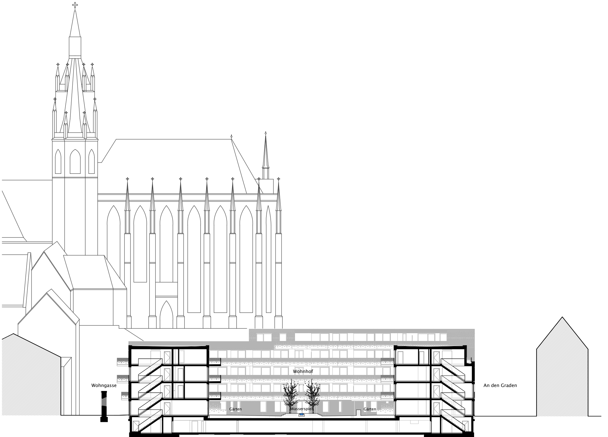
SCHNITT WOHNHOF
