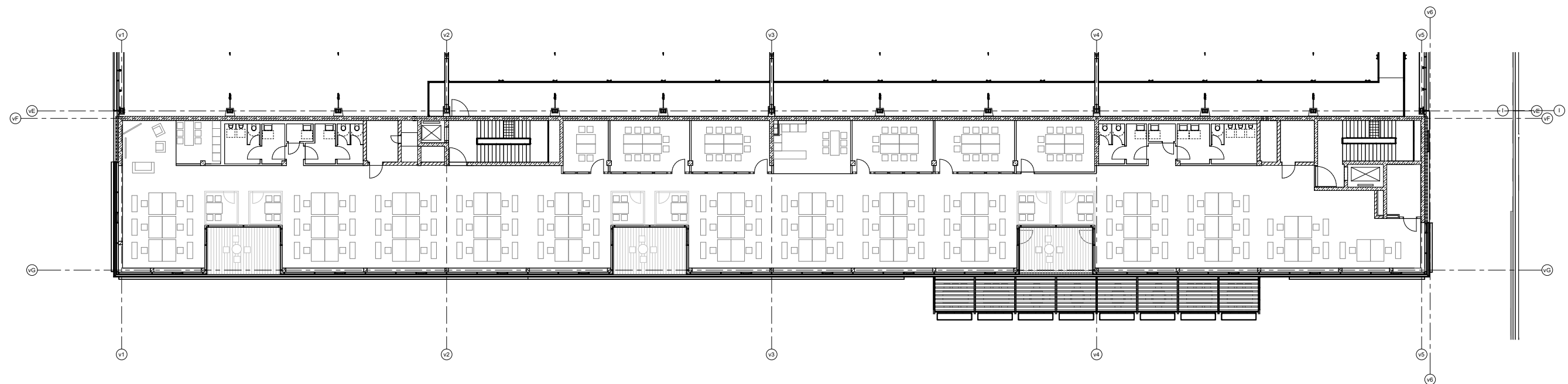
2. Obergeschoß
