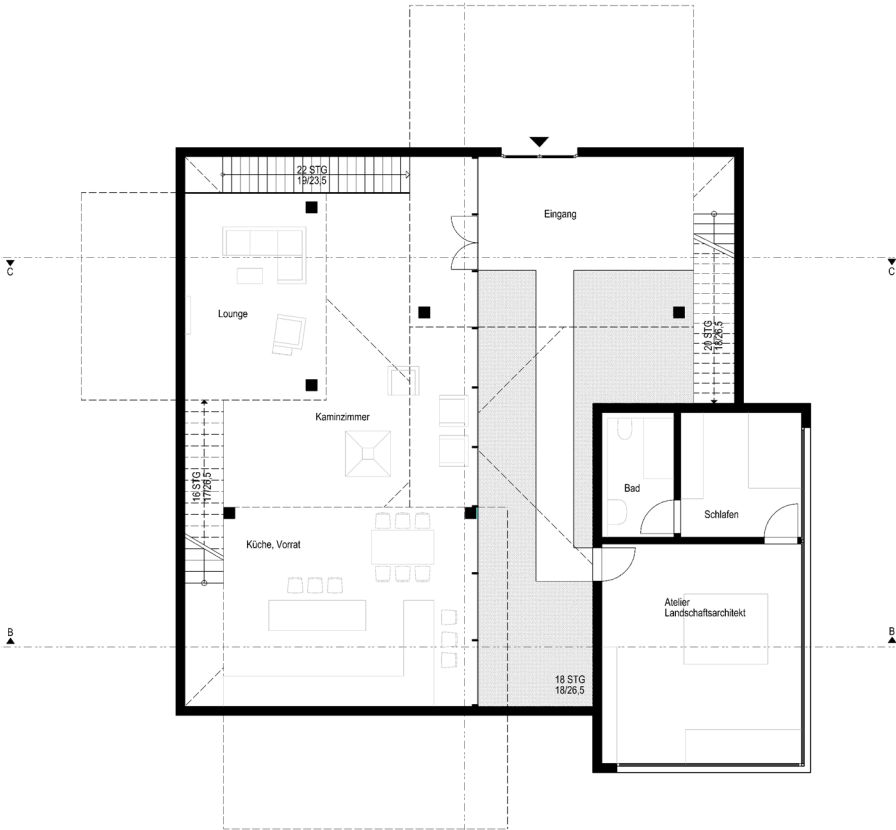
Erdgeschoss
