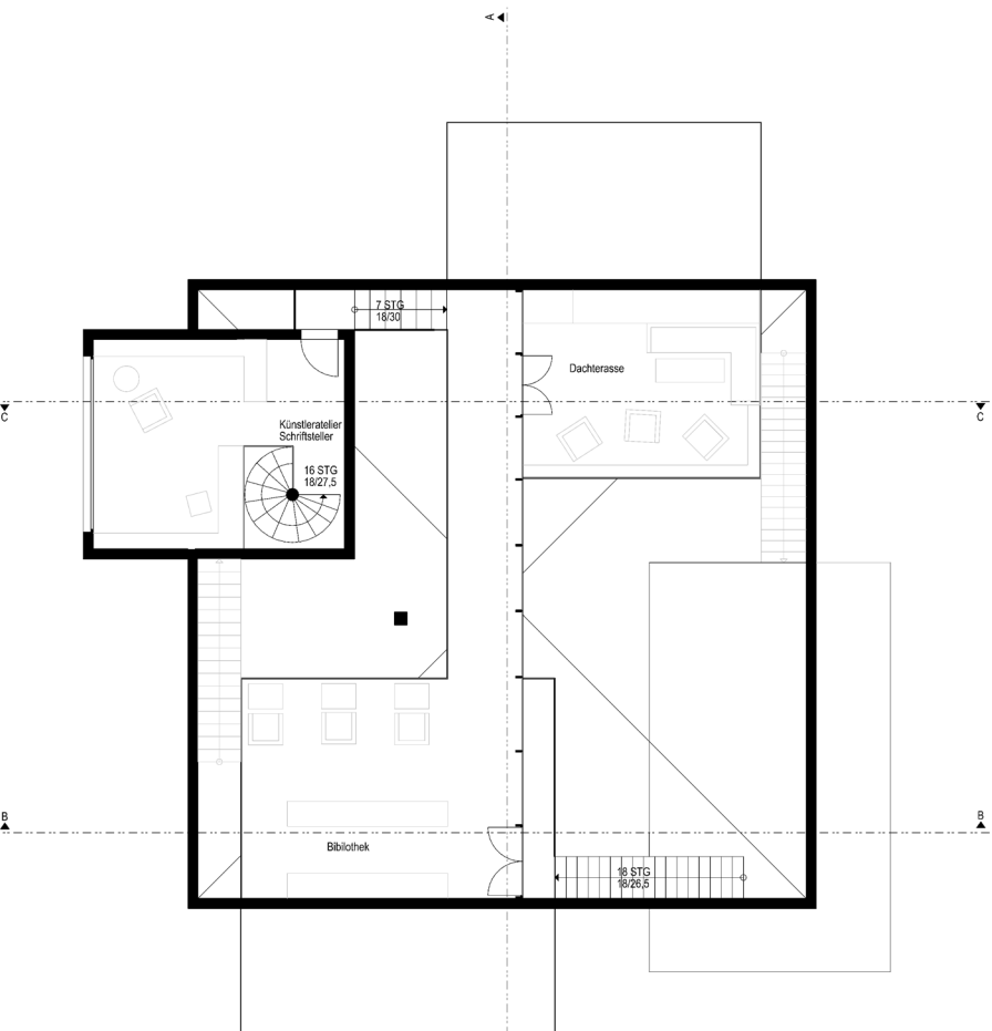
2. Obergeschoss
