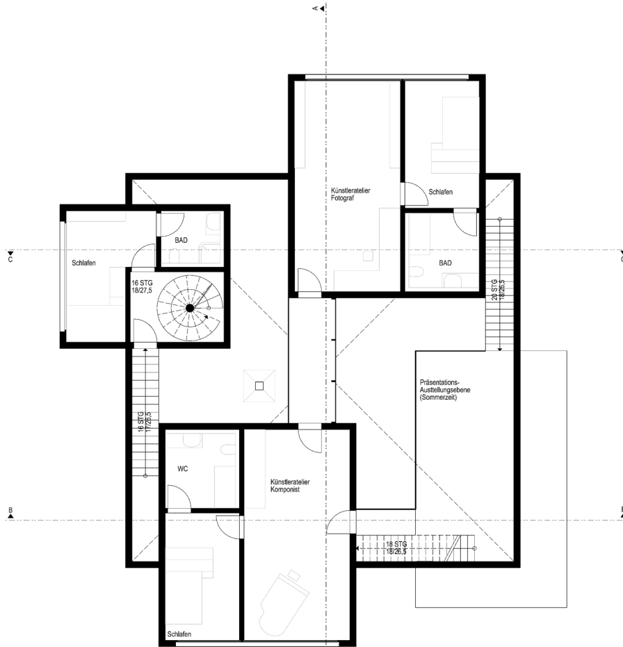
1. Obergeschoss
