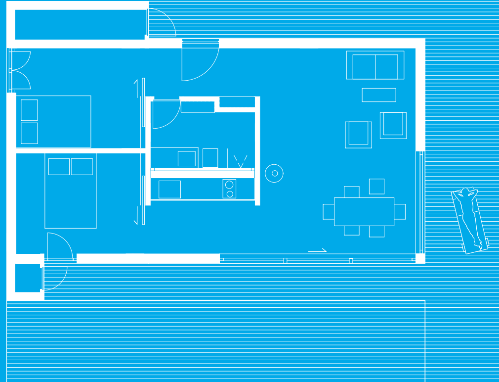
PIU 65 Grundriss | M 1:100
