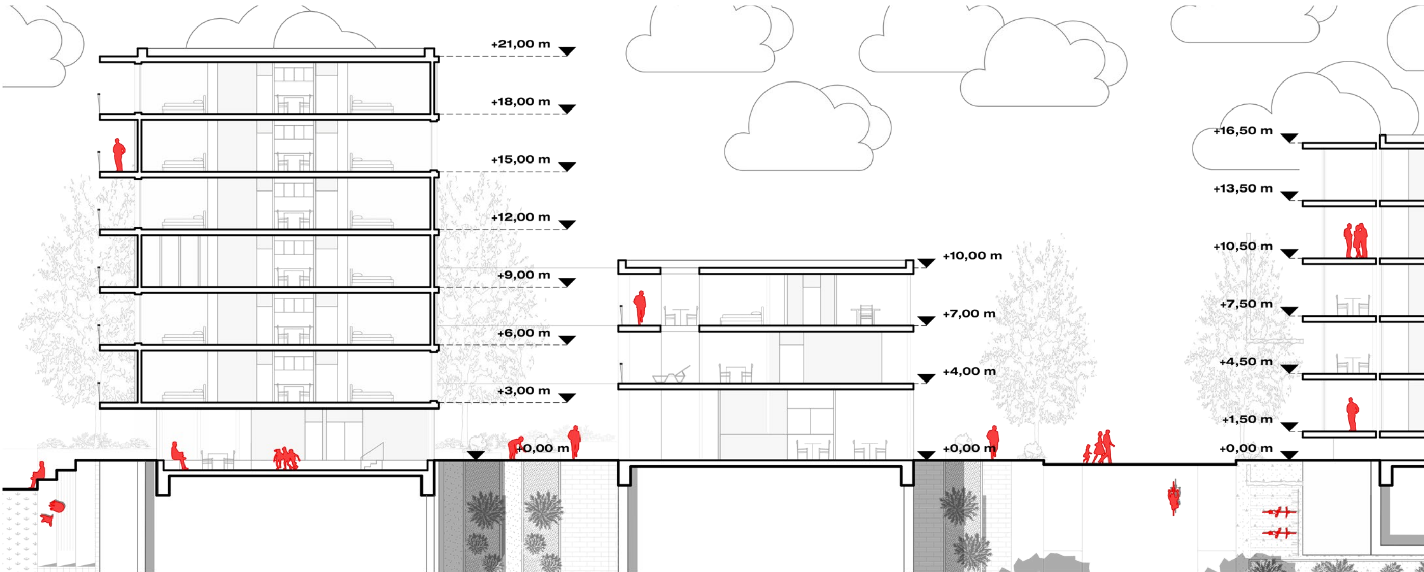
Schnitt Tafel 1 zu 200
