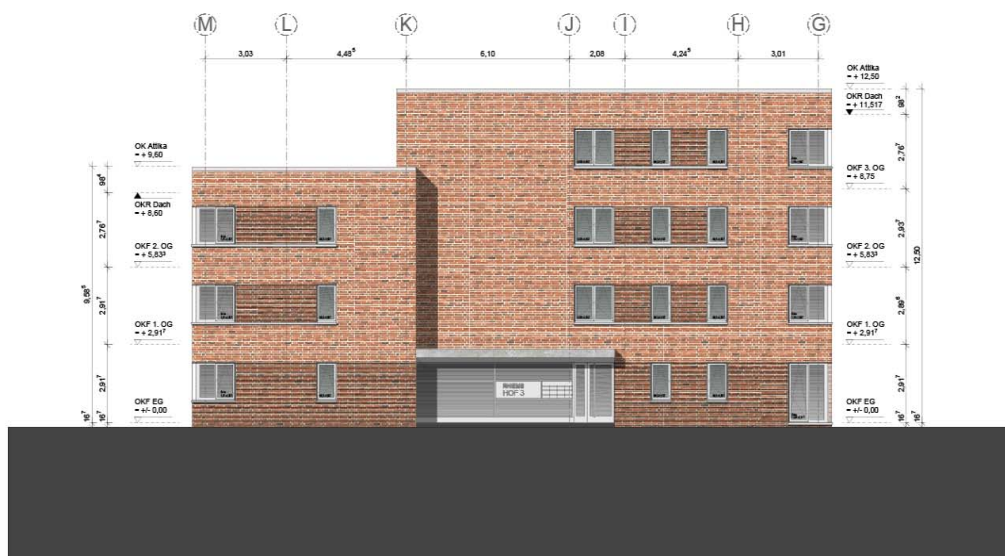
Abwicklung BK 2: Fassade Ost
