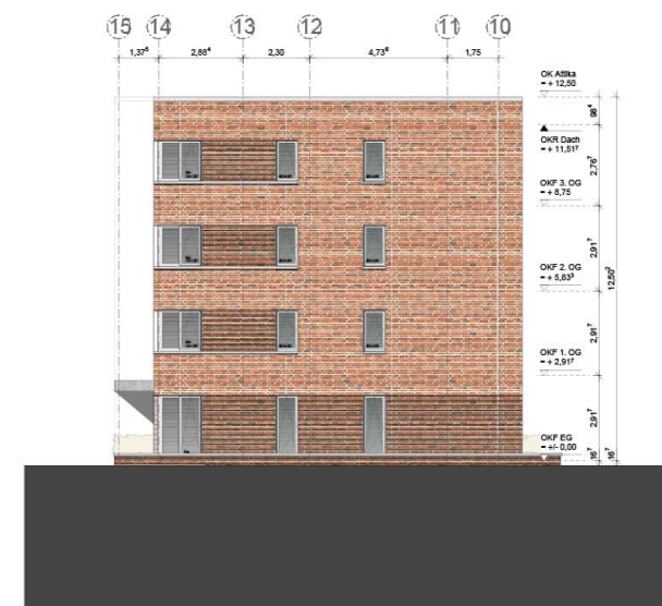
Abwicklung BK 2: Fassade Nord
