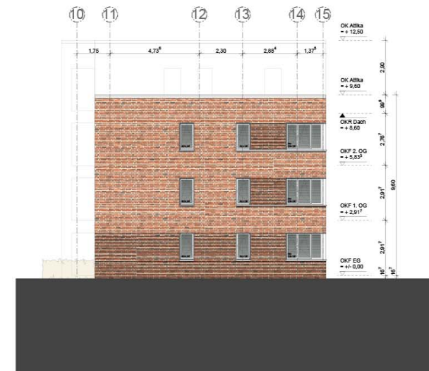
Abwicklung BK 2: Fassade Süd
