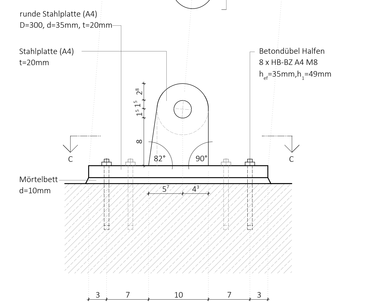
Schnitt D-D
