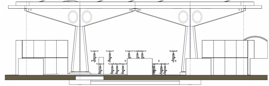
ANSICHT OST
