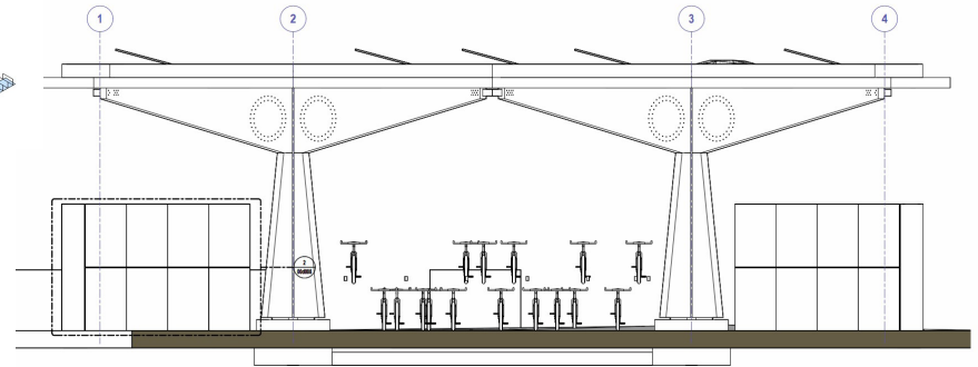
ANSICHT WEST
