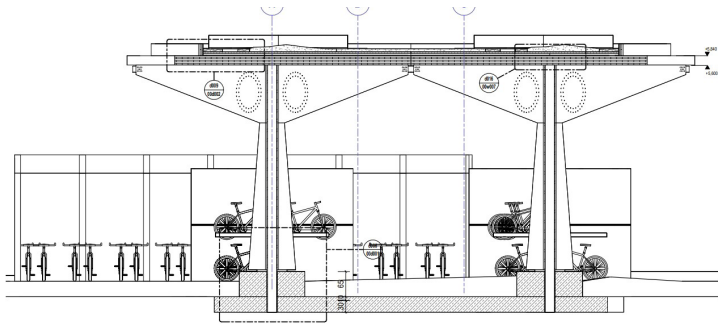
ANSICHT SÜD
