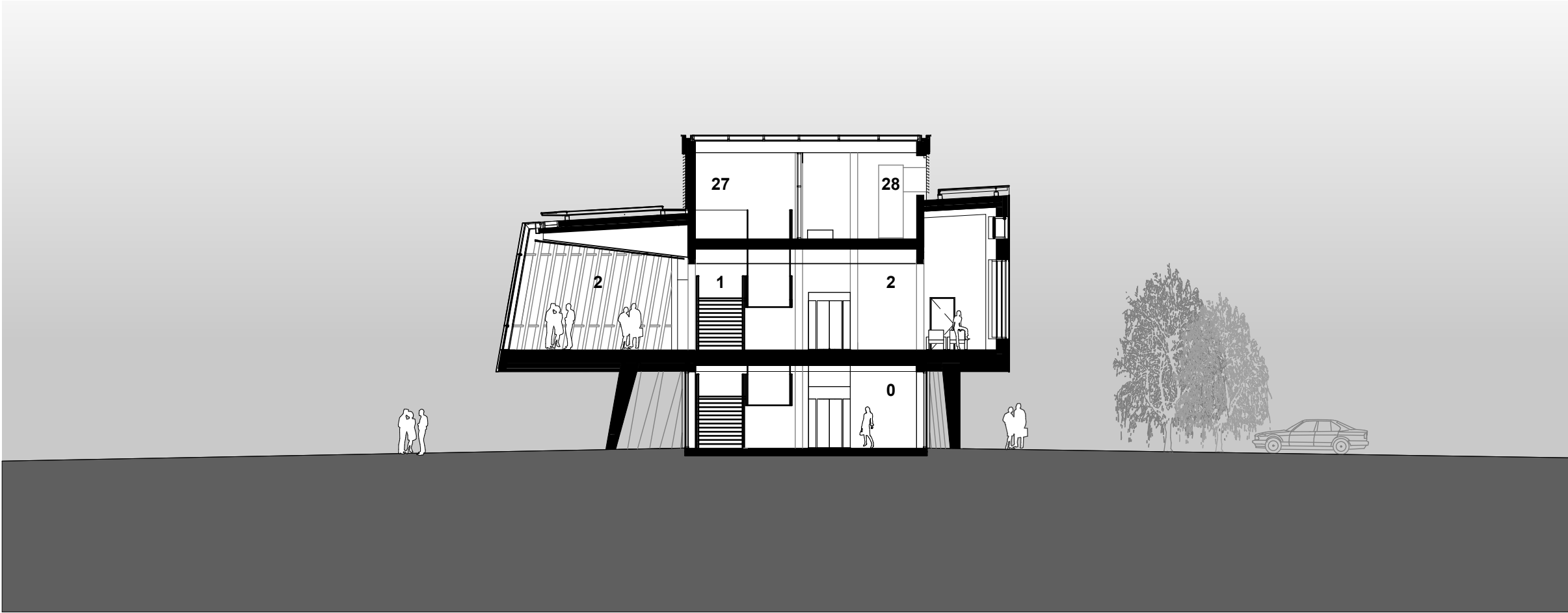
Querschnitt
