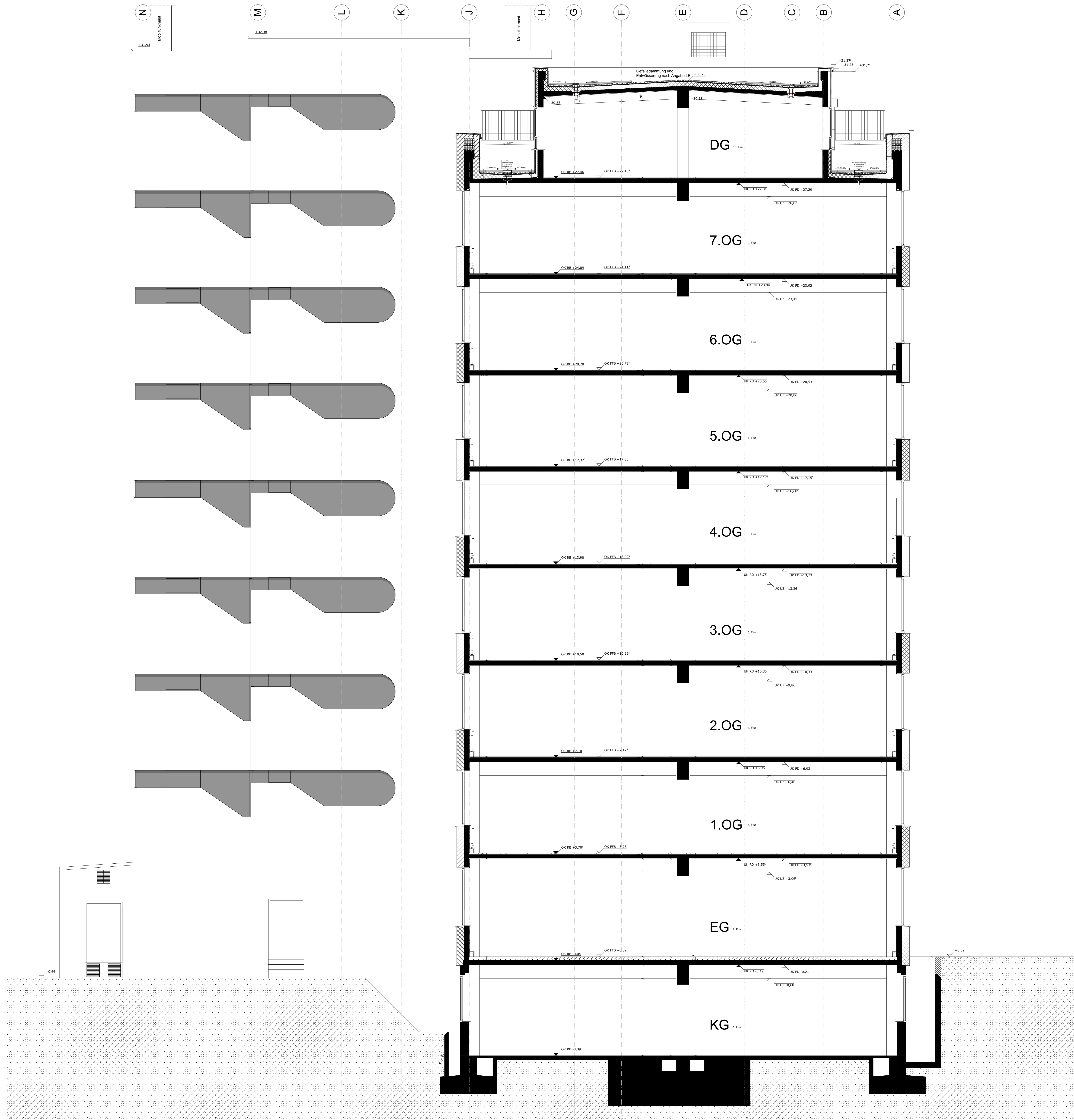
Schnitt B-B
