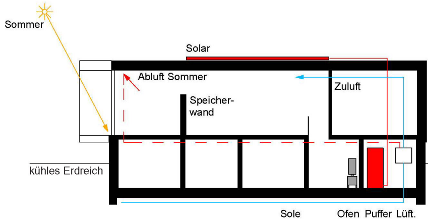
Prinzip Sommer
