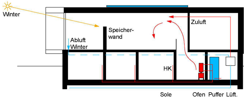
Prinzip Winter
