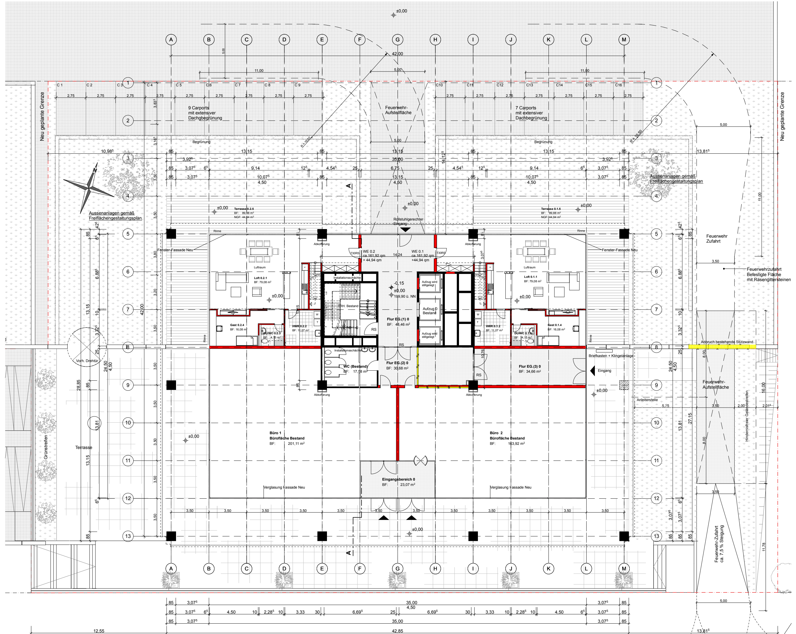
ERDGESCHOSS
