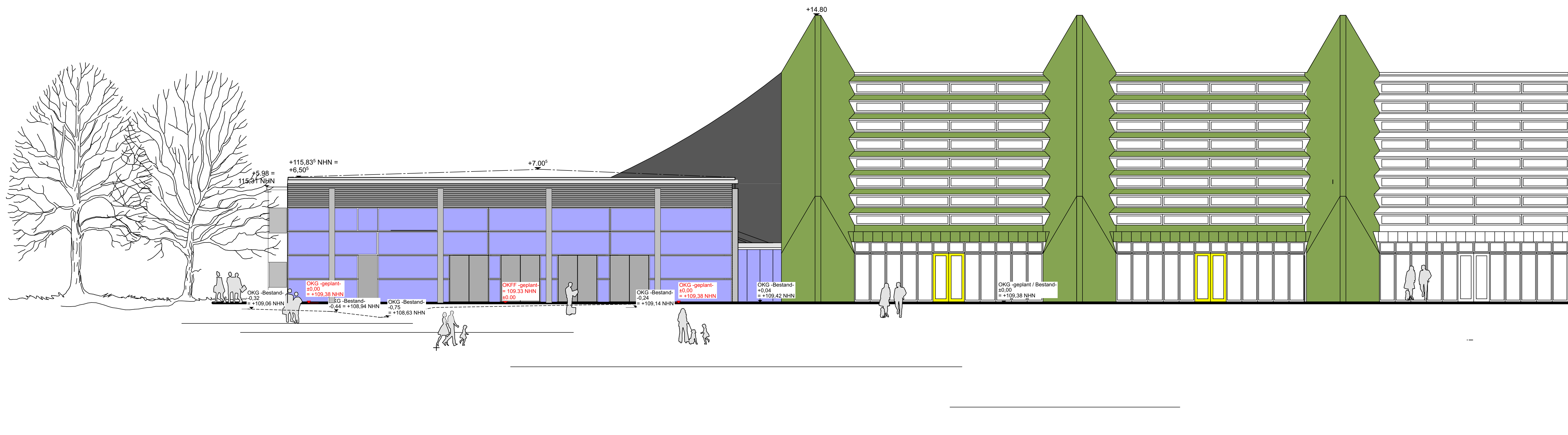
Ansicht Nord
