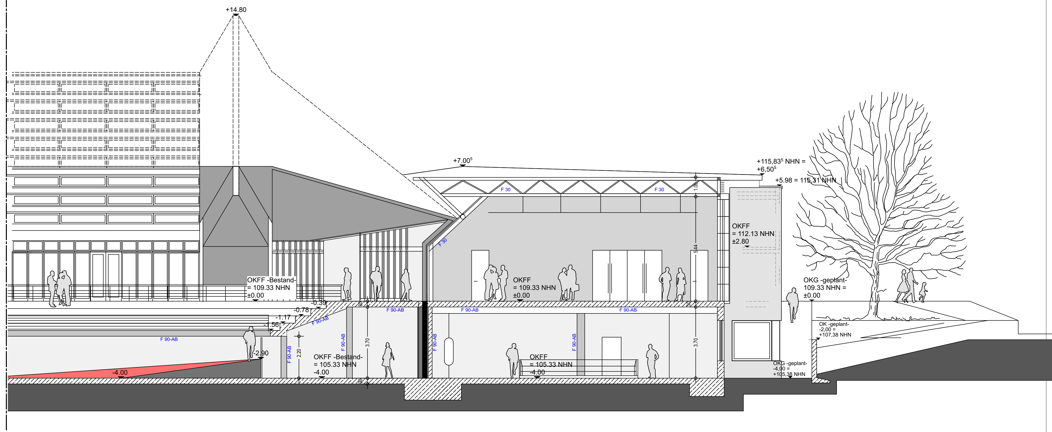
Schnitt Neubau A-A
